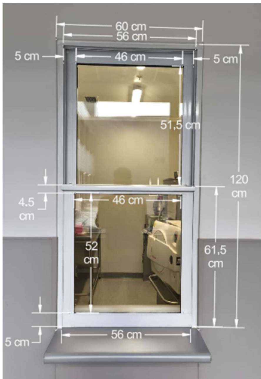
Ilustración 7 ventana guillotina referencial
